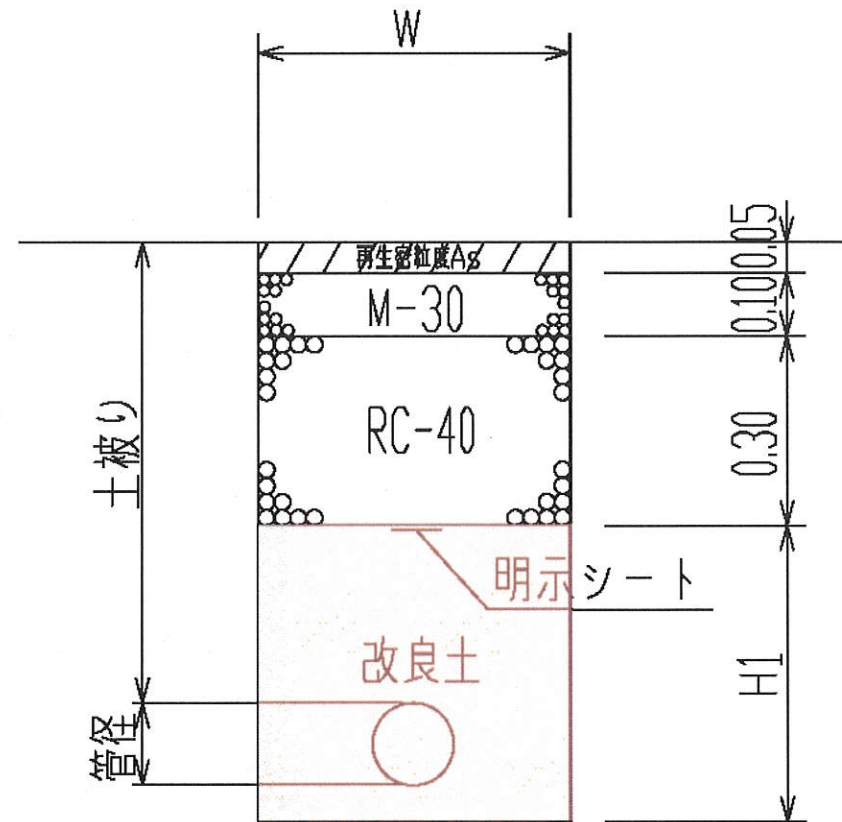
断面図
